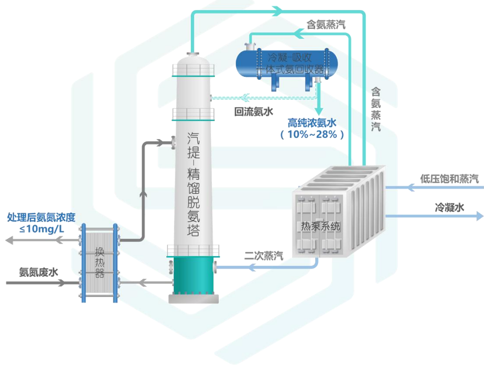
工艺流程示意图
