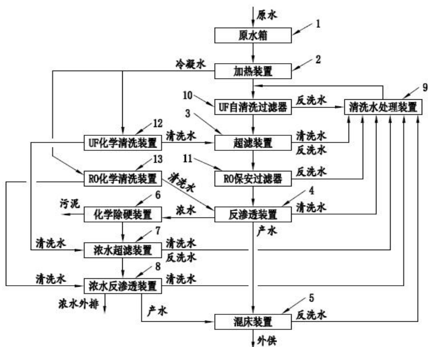
工艺流程示意图
