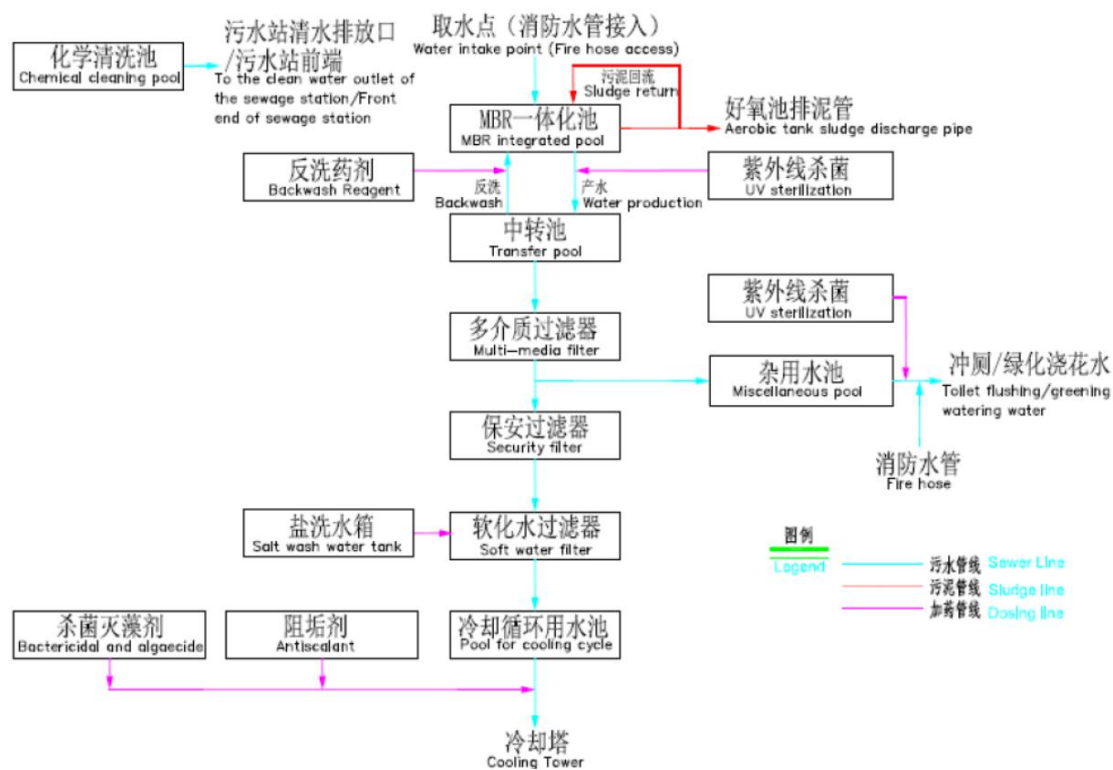
工艺流程示意图
