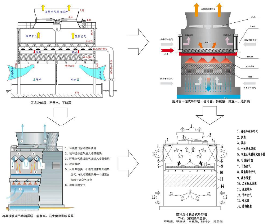
结构示意图
