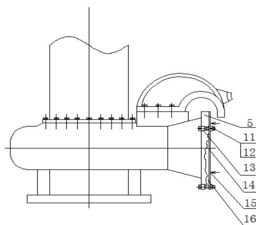
旋流井提升泵端面修复示意图
