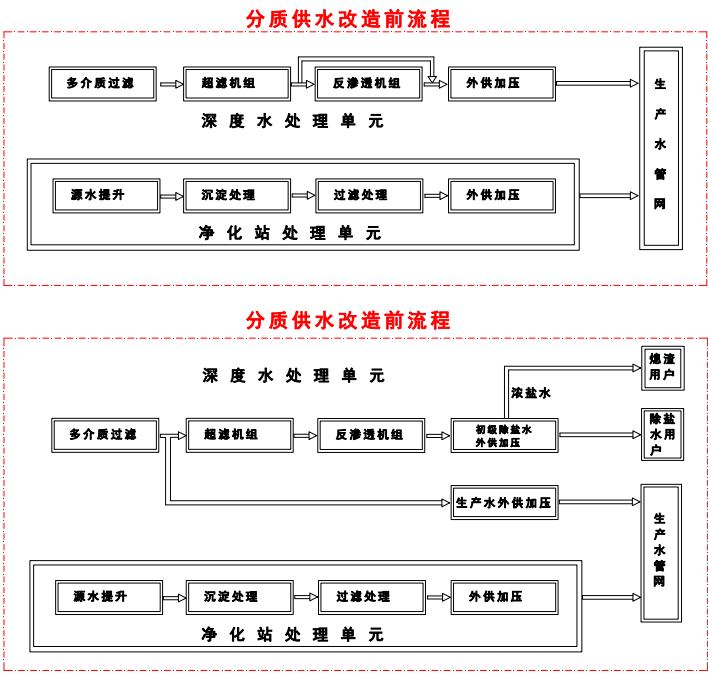
分质供水流程图
