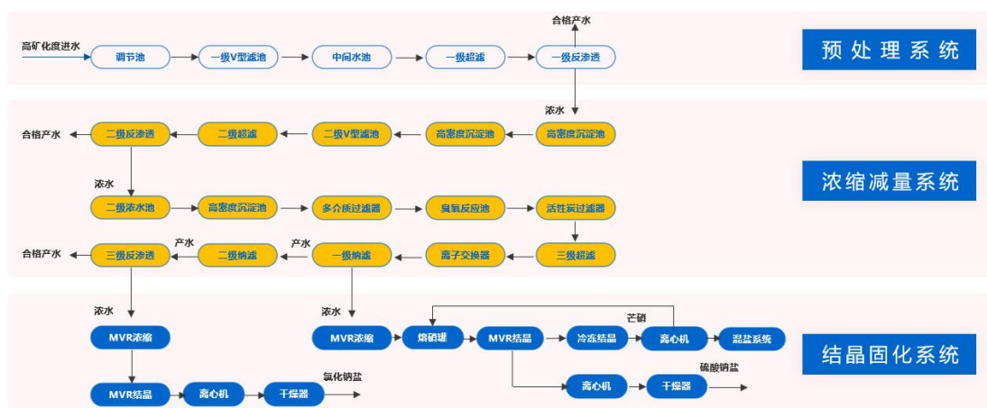
工艺路线图
