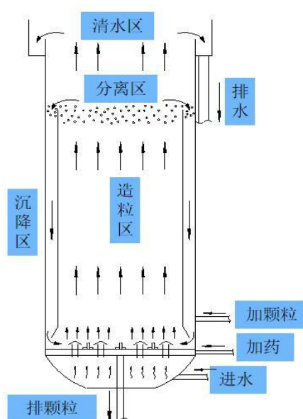
结构示意图
