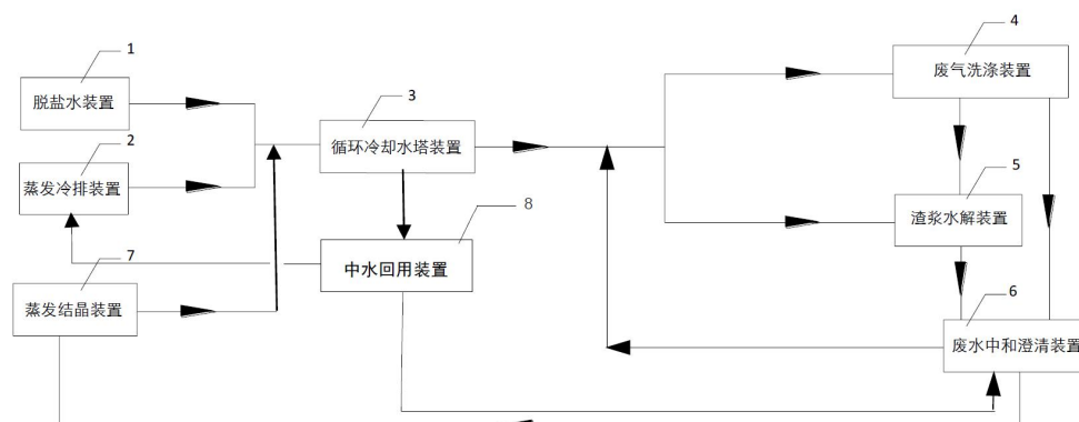
工艺流程示意图
